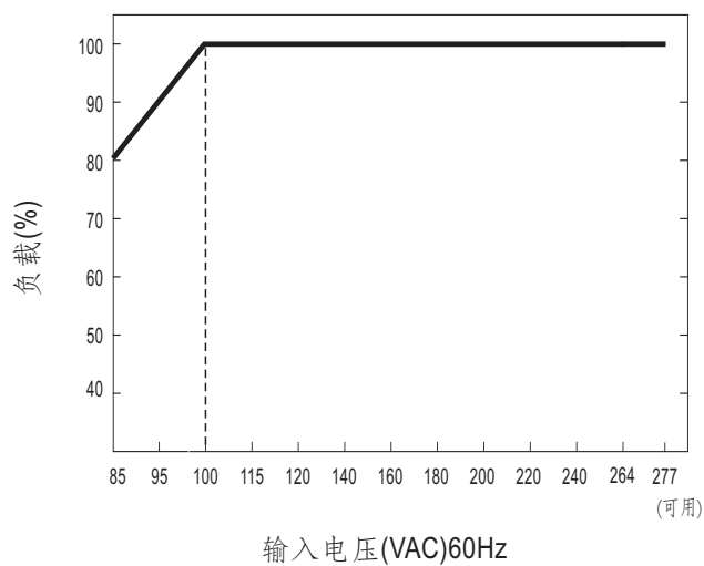
■ 减额输出VS输入电压曲线
