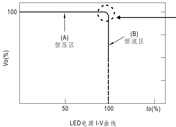
LED电源 I-V曲线
