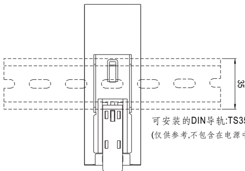
背面图
