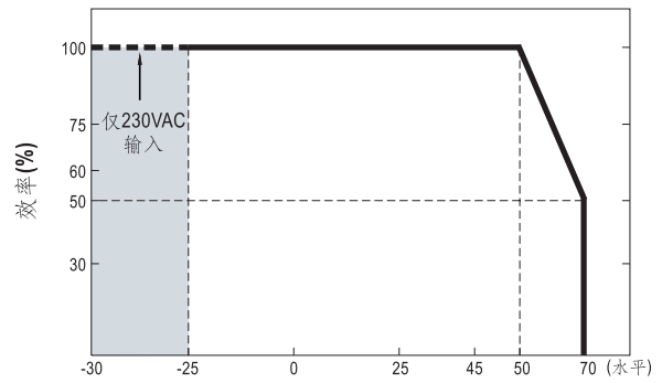
有2个CFM风扇水冷却系统的环境温度(°C)
